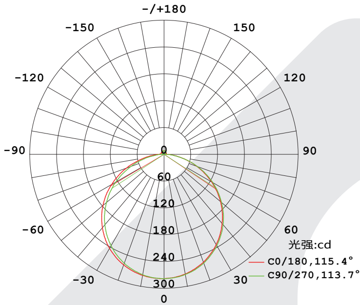
配光曲线
